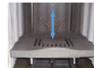
Rejilla de fuego de fundición regulable
